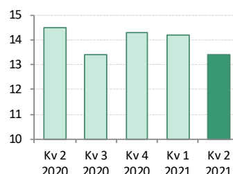
Kärnprimärkapitalrelation
